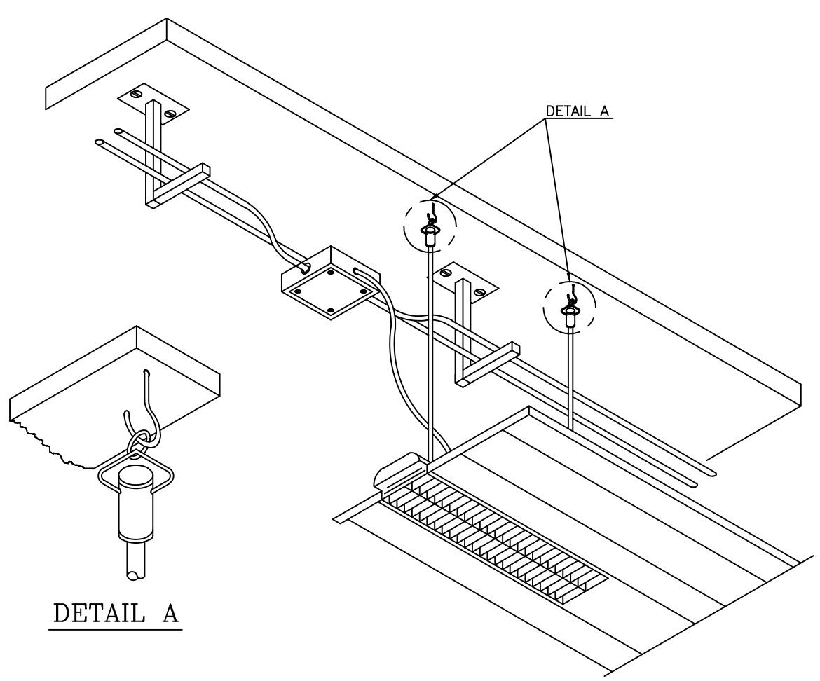
نحوه نصب چراغهای فلورسنت داخل سقف کاذب
