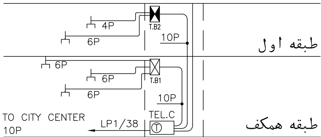
رایزر دیاگرام سیستم تلفن
