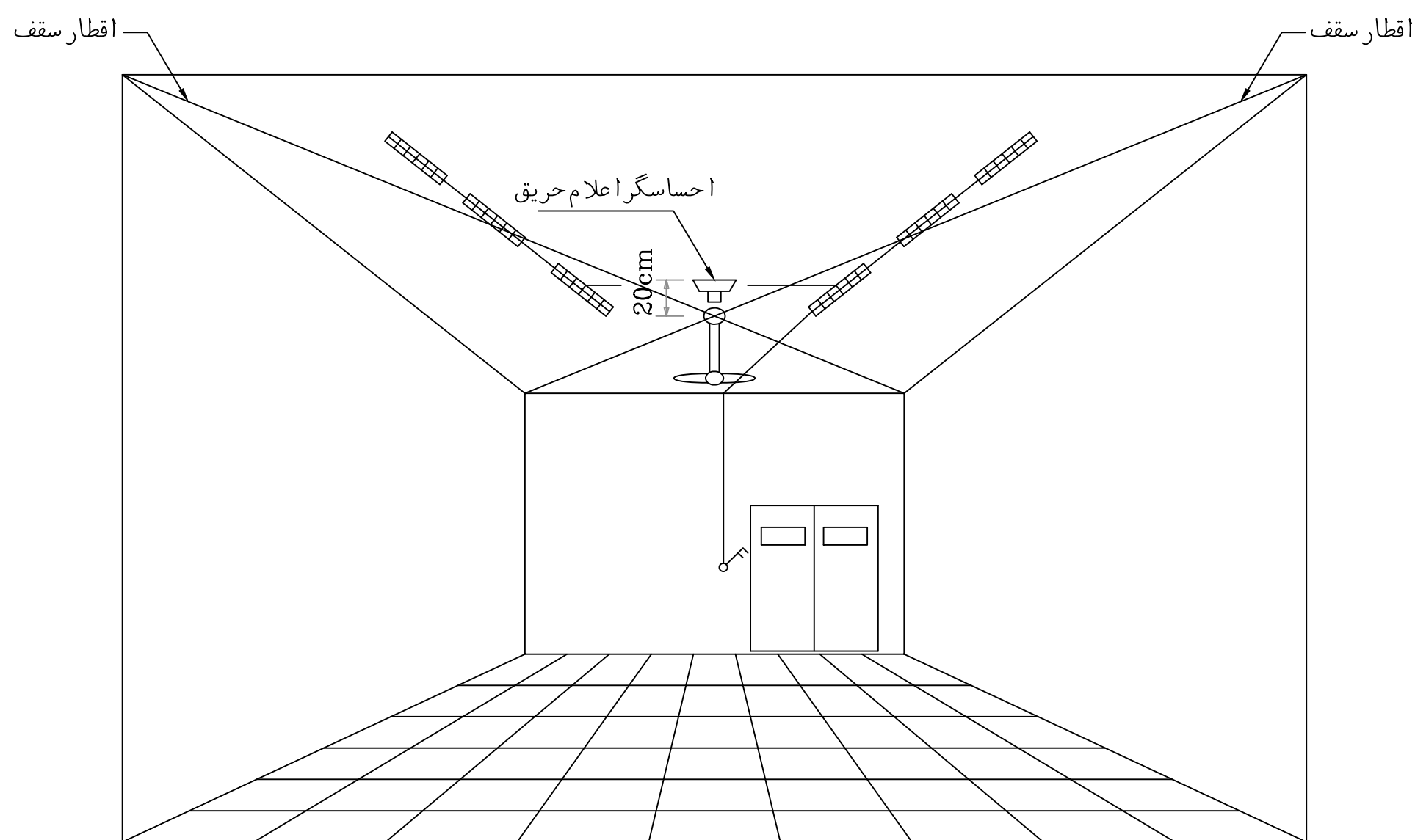
جزئیات اجرای لوازم برقی در سقف
