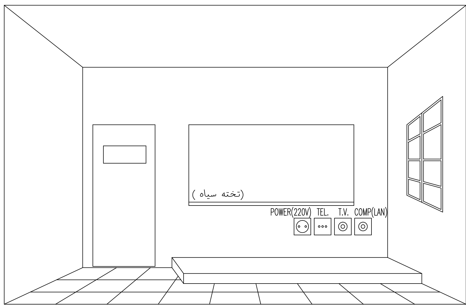
ترتیب اجرای پریزها در اتاق ها
