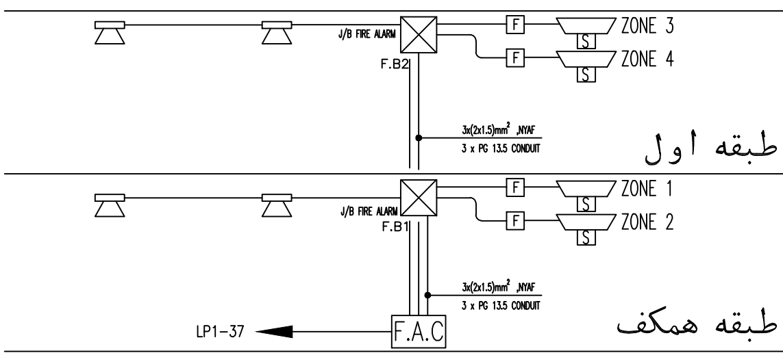
رایزر دیاگرام سیستم اعلام حریق
