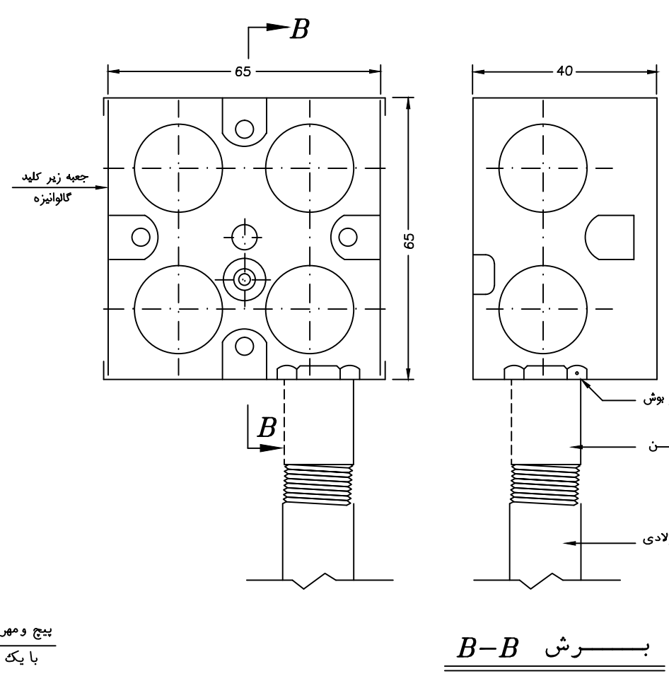
جزئیات اتصال جعبه کلید به لوله فولادی
