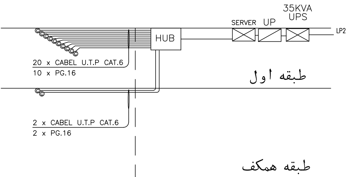
رایزر دیاگرام سیستم شبکه ارتباط محلی رایانه
