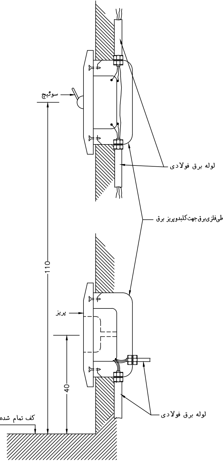
جزئیات نصب کلید و پریزهای برق
