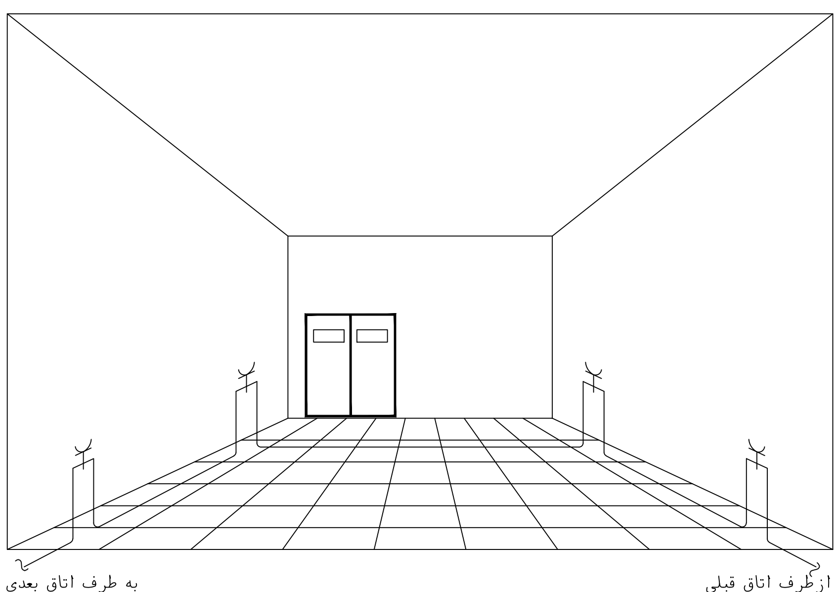
جزئیات اجرای سیستم پریزهای برق
