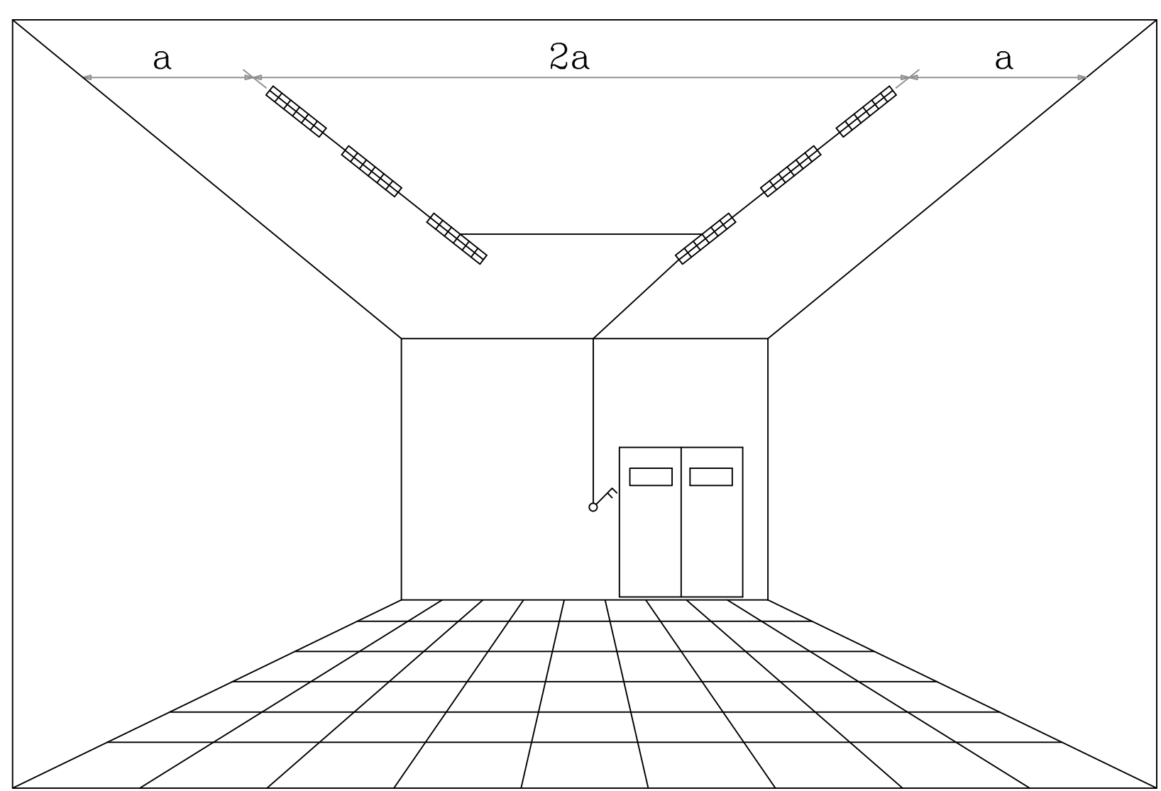
جزئیات اجرای سیستم روشنایی
