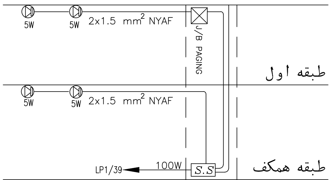
رایزر دیاگرام سیستم بلندگو
