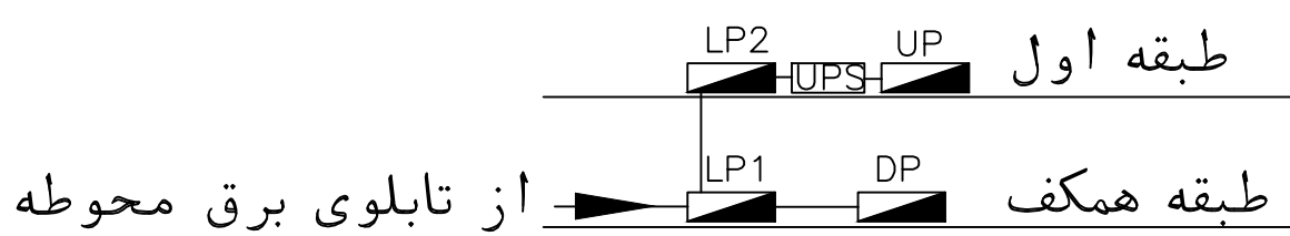
رایزر دیاگرام سیستم برق رسانی
