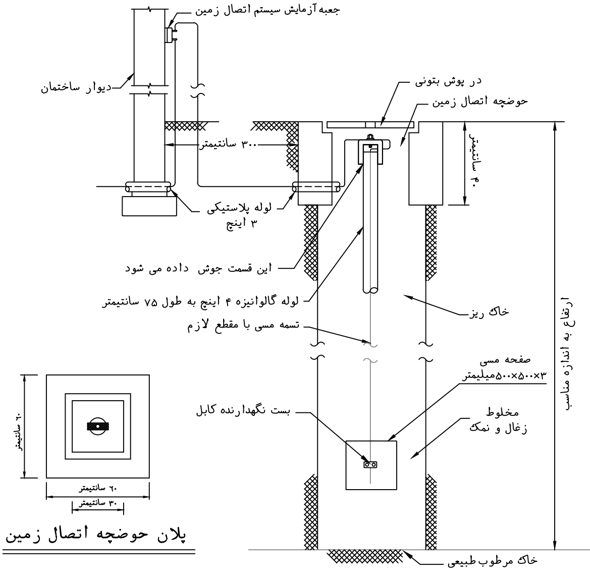
جزئیات نصب سیستم اتصال زمین با الکتروود صفحه مسی
